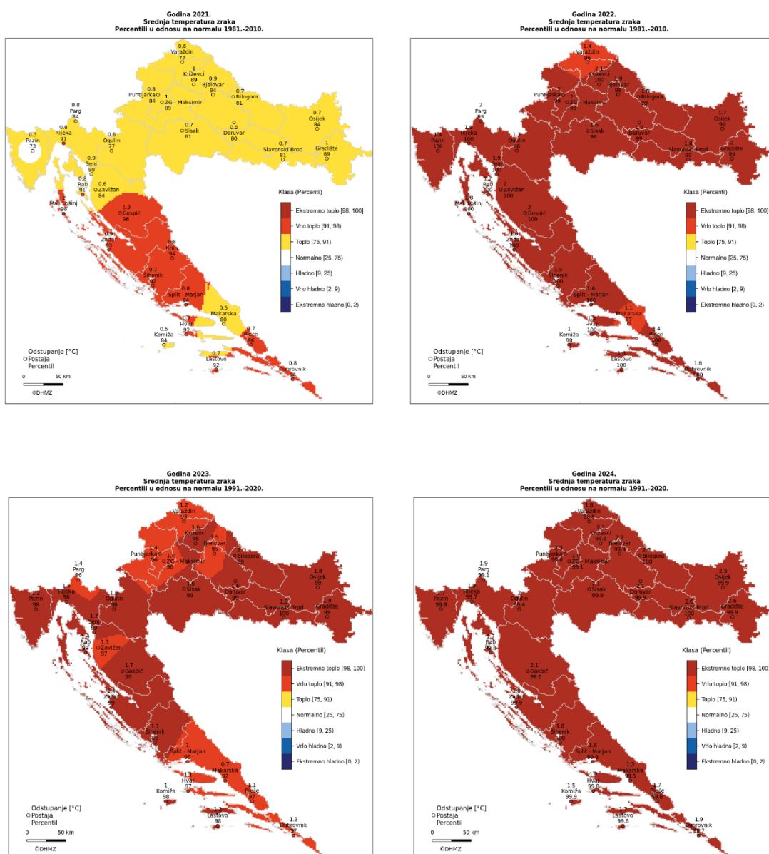
Slika 2.1-2 Odstupanja srednje godišnje temperature zraka [°C] za 2021. i 2022. od prosjeka razdoblja 1981. – 2010., te odstupanja srednje godišnje temperature zraka [°C] za 2023. i 2024. od prosjeka razdoblja 1991. – 2020.
