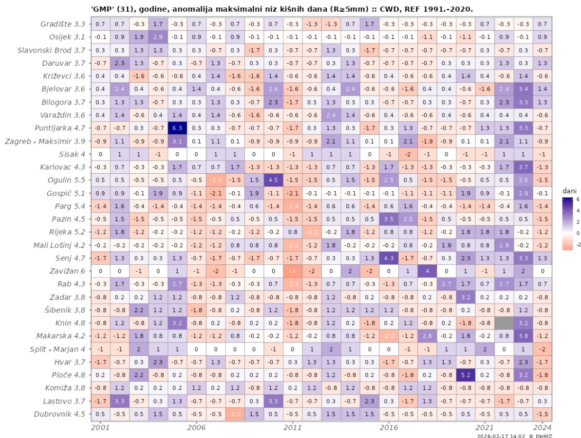
Slika 4.4-1 Odstupanja maksimalne duljine kišnih razdoblja od prosjeka razdoblja 1991. – 2020. tijekom 2001. – 2024. Prosječne duljine maksimalnih nizova kišnih dana razdoblja 1991. – 2020. naznačene su brojem kraj naziva meteorološke postaje.
