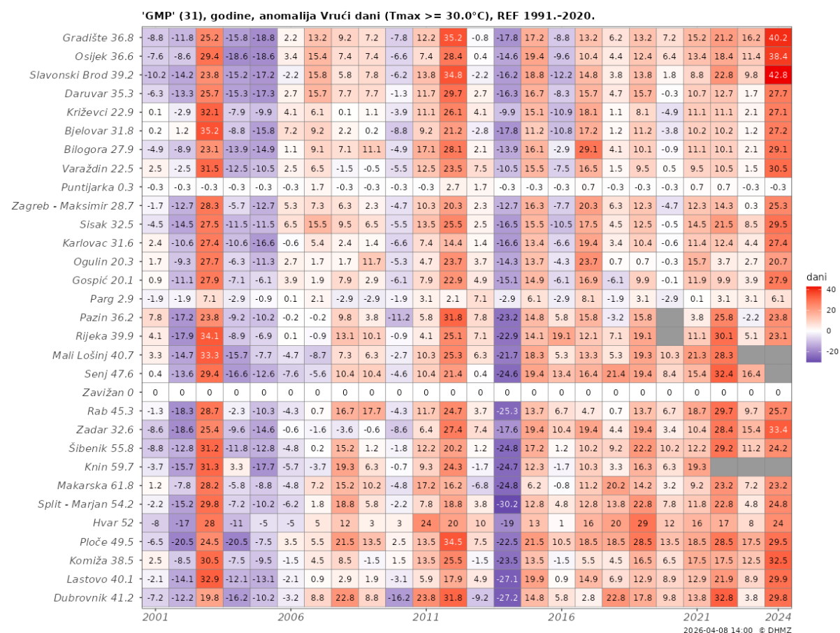
Slika 2.2.-1 Odstupanja godišnjeg broja vrućih dana od prosjeka razdoblja 1991. – 2020. tijekom 2001. – 2024. Prosječni broj vrućih dana u razdoblju 1991. – 2020. naznačen je brojem kraj naziva meteorološke postaje.
