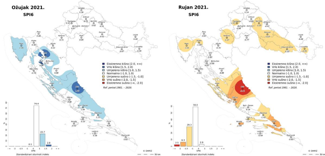
Slika 4.2-1 Standardizirani oborinski indeks, SPI6 za ožujak (lijevo) i rujan (desno) 2021. godine u odnosu na prosjek razdoblja 1981. – 2020.
