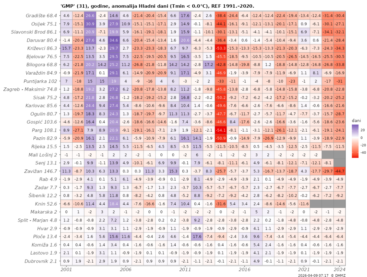
Slika 2.3-1 Odstupanja godišnjeg broja hladnih dana od prosjeka razdoblja 1991. – 2020. tijekom 2001. – 2024. Prosječni broj hladnih dana u razdoblju 1991. – 2020. naznačen je brojem kraj naziva meteorološke postaje.
