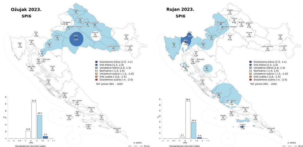
Slika 4.2-5 Standardizirani oborinski indeks, SPI6 za ožujak (lijevo) i rujan (desno) 2023. godine u odnosu na prosjek razdoblja 1981. – 2020.
