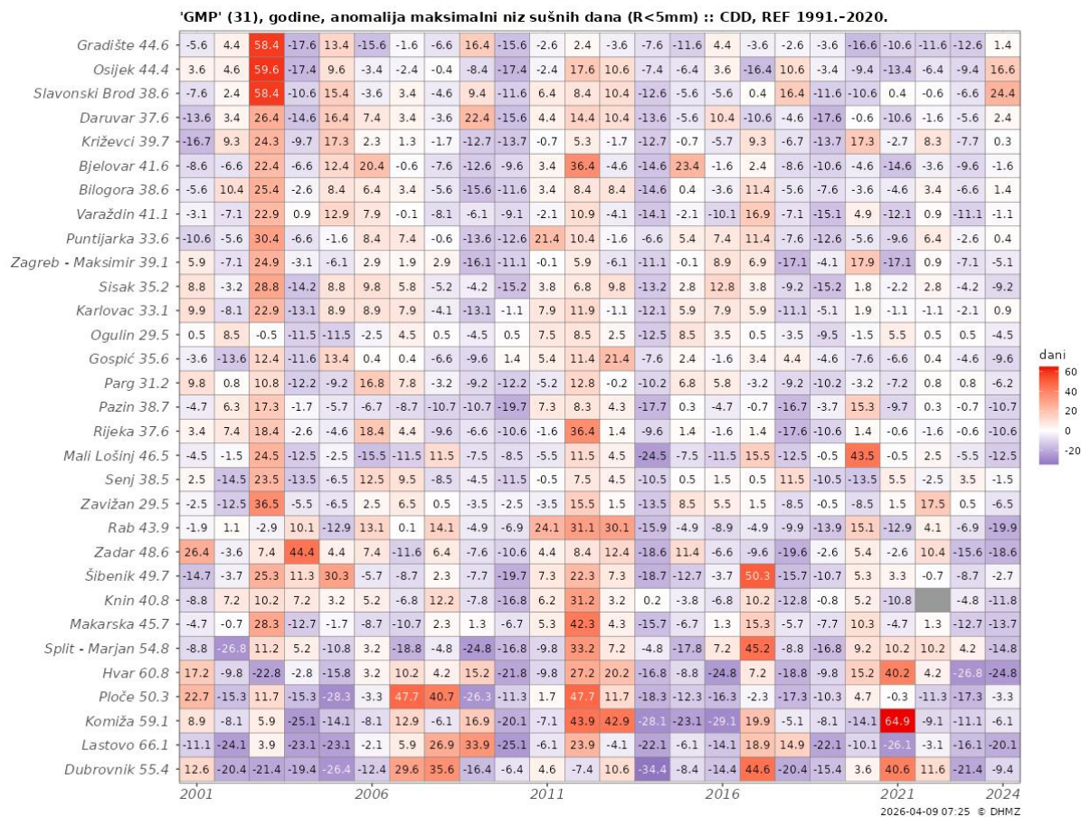
Slika 4.3-1 Odstupanja maksimalne duljine sušnih razdoblja od prosjeka razdoblja 1991. – 2020. tijekom 2001. – 2024. Prosječne duljine maksimalnih nizova sušnih dana razdoblja 1991. – 2020. naznačena su brojem kraj naziva meteorološke postaje.
